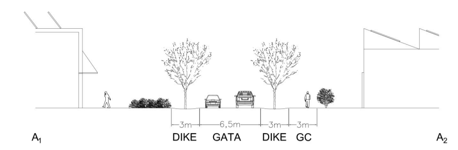
SEKTION A 1 -A 2 , Verksamhetsgata "Slingan"
