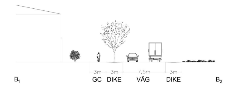
SEKTION B 1 -B 2 , Åkeshögsvägen
