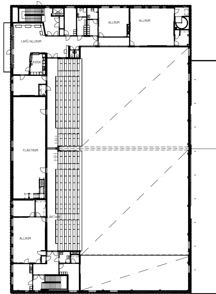
IDROTTSHALL - PLAN 2
